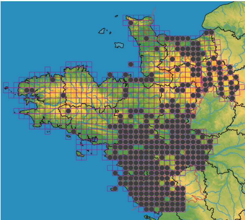
Carte 1 : Carte de répartition de Rubus caesius L. à la maille UTM 10x10km toutes périodes confondues (base de données Calluna du CBN Brest)
