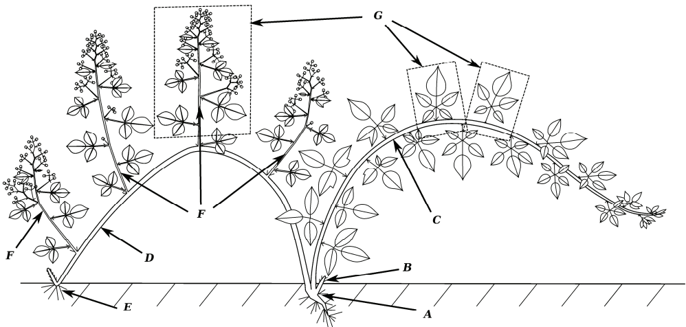
Figure 1 : Structure générale d'un Rubus à tiges bisannuelles capables de marcottage (cas le plus fréquent).
